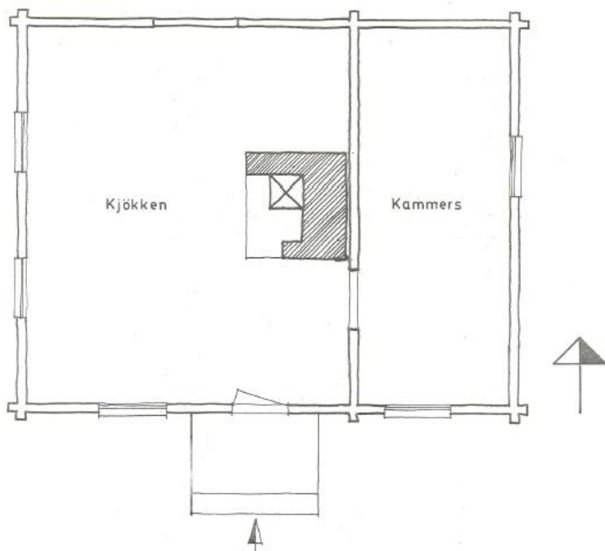
Skomakerstua på Veset. Eksempel på grunnplan, akershusisk stuetype. Oppmåling Jan Erik Horgen 1976.
