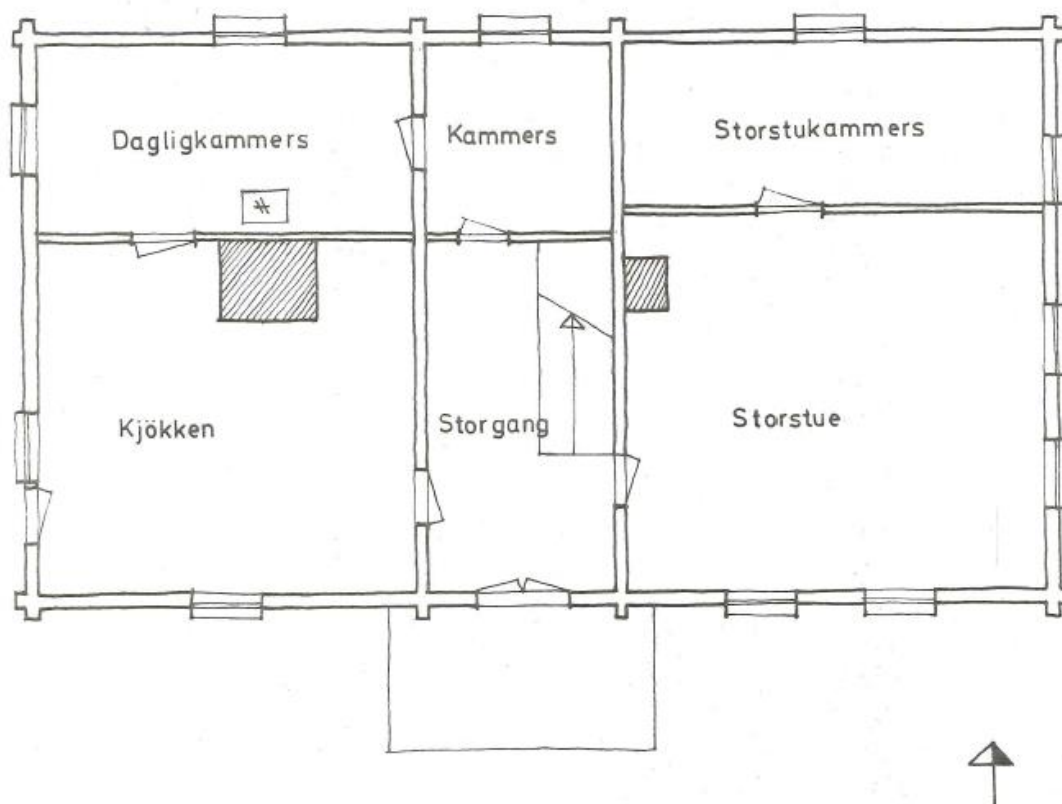
Hovedbygningen på Strøm i Fenstad. Eksempel på grunnplan, midtkammerbygning. Oppmåling Jan Erik Horgen 1975.
